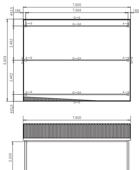
■ 3台用 構造仕様図面より 品番「30-7960/10」
