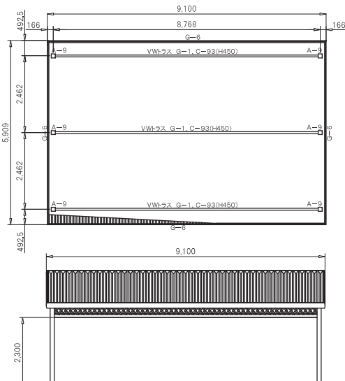
■ 3台用+駐輪場用 構造仕様図面より 品番「30-9160/10」
