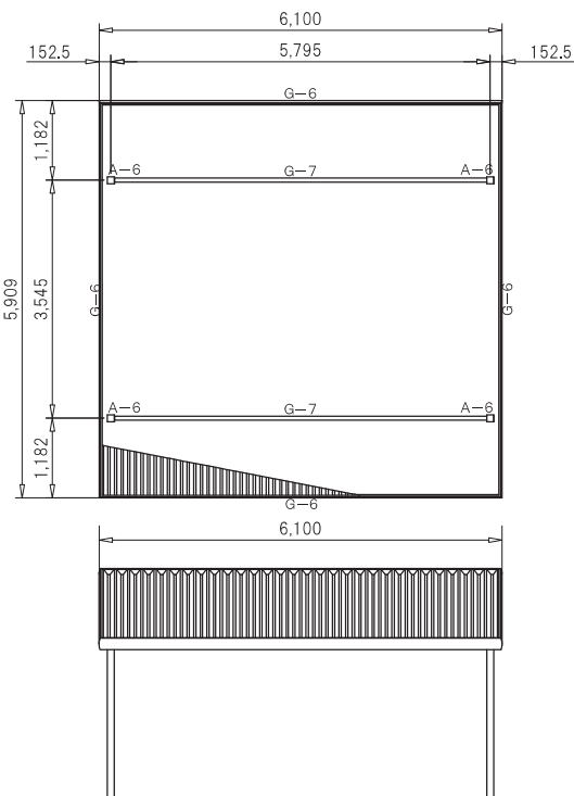
構造仕様図面より 品番「50-6160/10」
